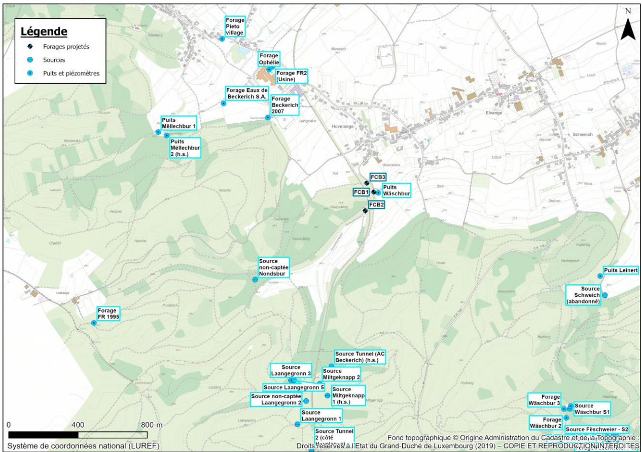
Figure 9. Localisation des puits, captages et forages à proximité du site d'étude
