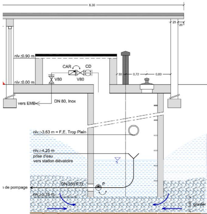
Figure 6. Coupe technique du captage Wäschbour (Source : Dossier de délimitation ZPS non-publié)
